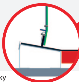
* Kónicky otevřené utěsnění okrajů pomocí kluzných pásových snosů bez prostupu (pohled ve směru dopravy)
