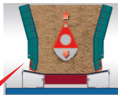
* Kónicky otevřené utěsnění okrajů pomocí kluzných pásových snosů bez prostupu (pohled ve směru dopravy)
