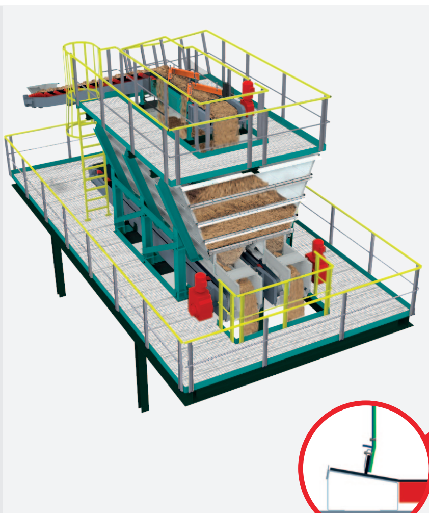
* Dvojitý zásobník s vynášecími pásovými dopravníky
