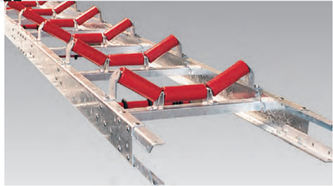
* Das Bandgestell als C-Gestell
